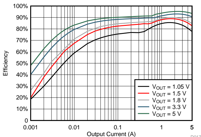
TPS565201 效率
