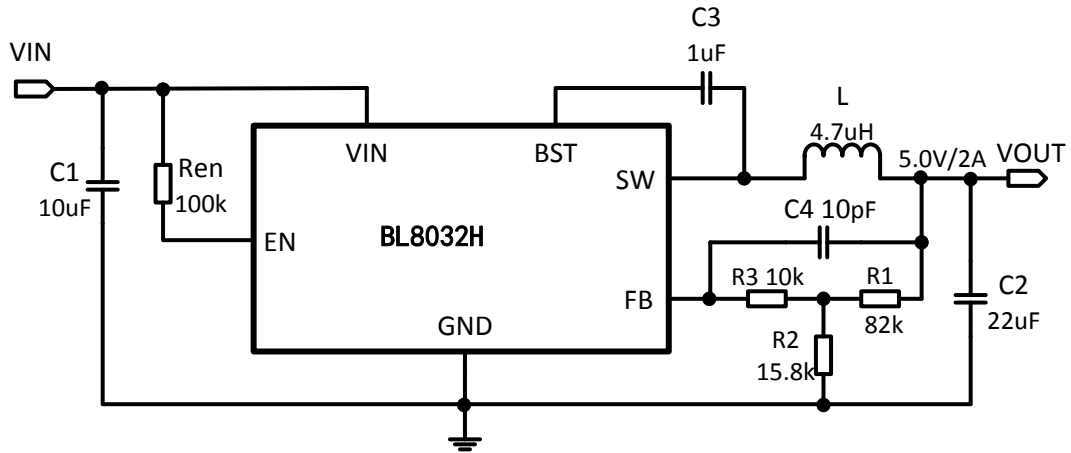
Figure3. 12V VIN, 5V/2A
