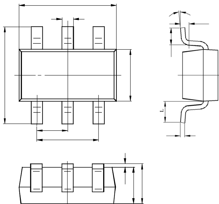
SOT23-6
