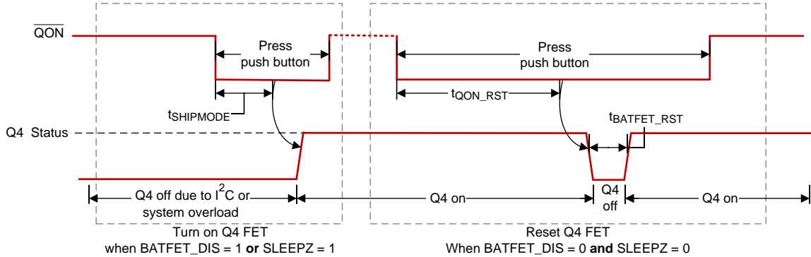
图 18. \overline{QON} Timing
