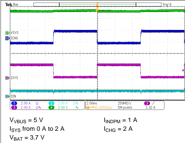
图 44. System Load Transient
