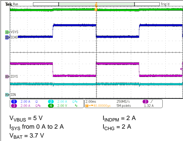
图 46. System Load Transient
