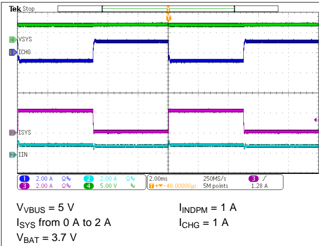
图 42. System Load Transient
