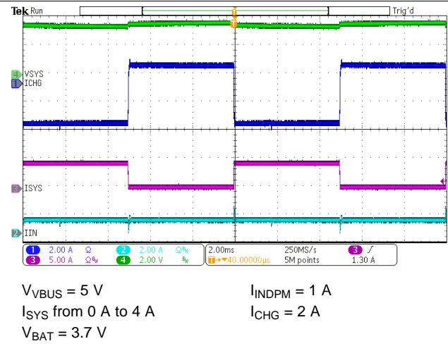
图 45. System Load Transient
