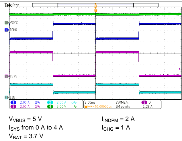
图 43. System Load Transient
