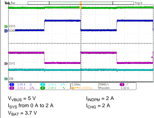
图 46. System Load Transient
