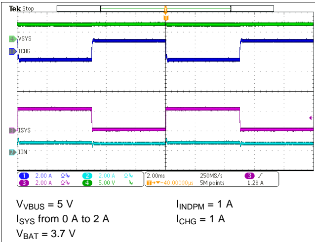
图 42. System Load Transient
