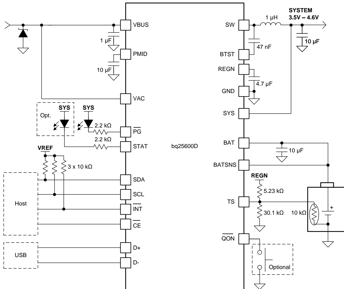
图 29. bq25600D Applications Diagram
