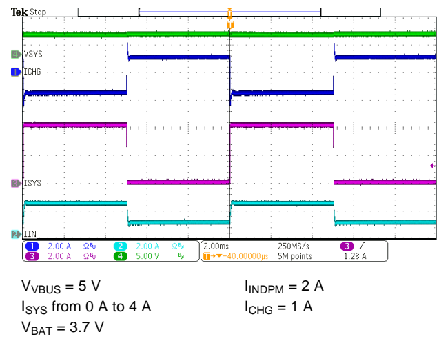
图 43. System Load Transient
