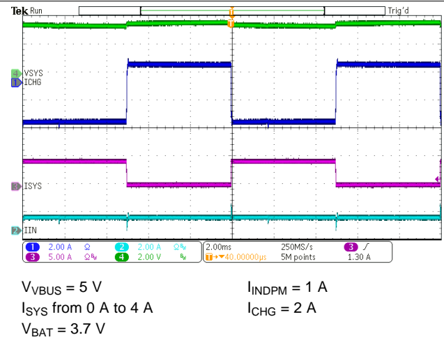
图 45. System Load Transient
