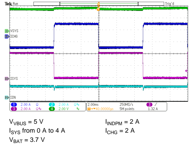
图 47. System Load Transient
