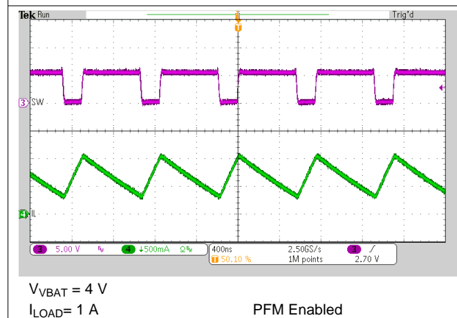
图 40. OTG Switching
