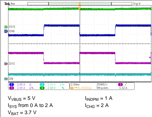
图 44. System Load Transient
