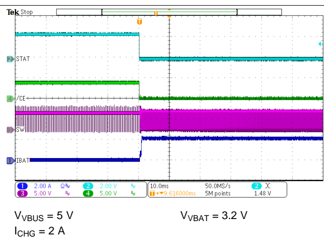
图 37. Charge Enable
