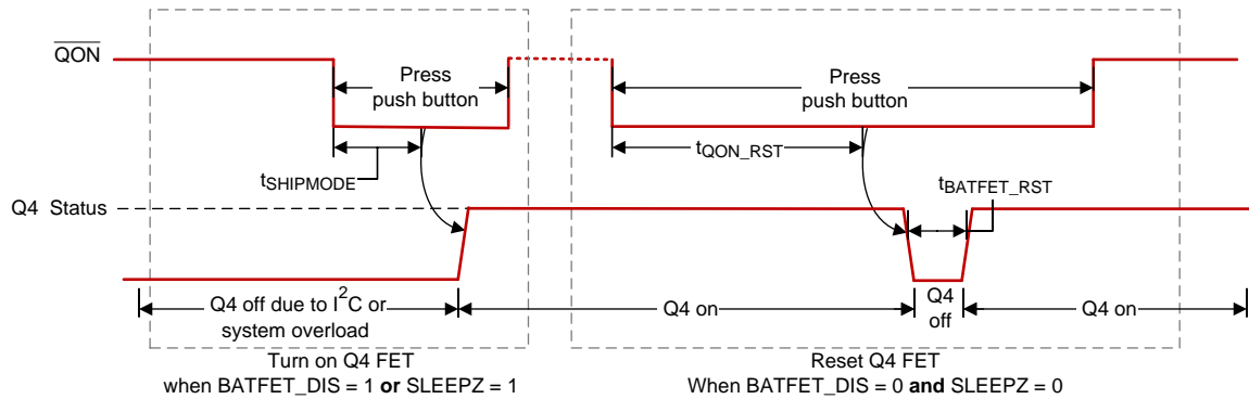
图 18. \overline{QON} Timing
