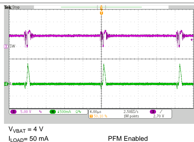
图 39. OTG Switching
