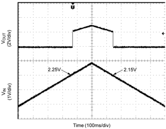
UVLO
