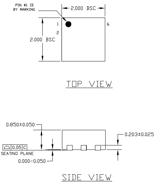
6 Pin 2mm x 2mm MLF ® (ML)
