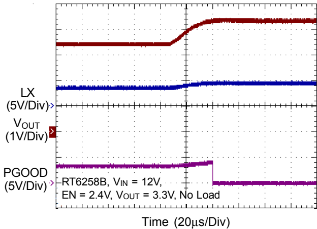
V_{OUT} OVP
