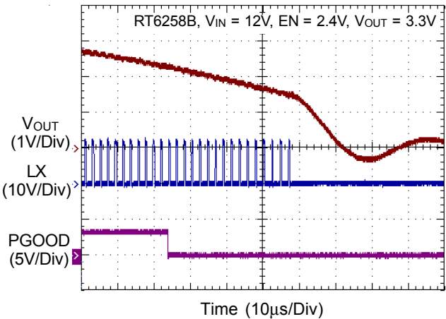
V_{OUT} UVP
